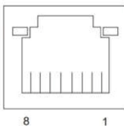
Slika 13. Priključak RJ45 (strana na kojoj je priključak)
