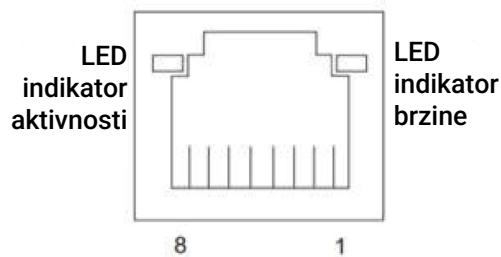
Slika 13. Priključak RJ45 (strana na kojoj je priključak)
