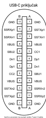
Slika 9. USB-C priključak
