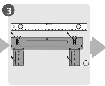
Postavite noseću pločicu
