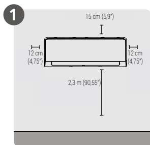
Odredite mesto ugradnje
