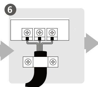
Povežite strujne instalacije (ne važi za neke lokacije u Severnoj Americi)
