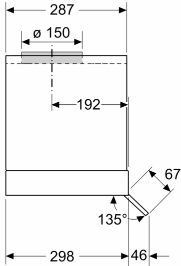
Dimenzije u mm Bočni prikaz
