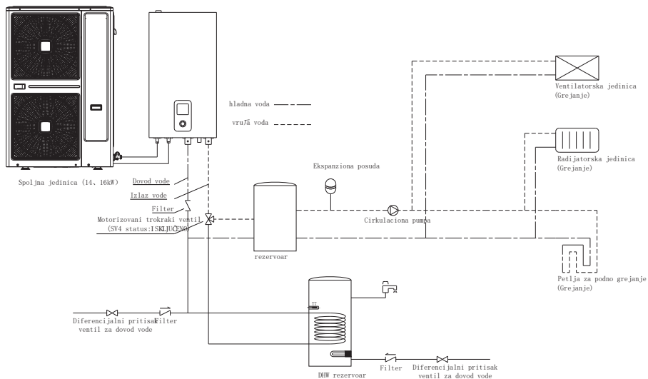
Slika 3.8 Rad u režimu grejanja (bez režima hlađenja)
