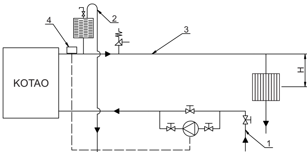
Slika 6.2 - sa nalegajućim cevnim termostatom
