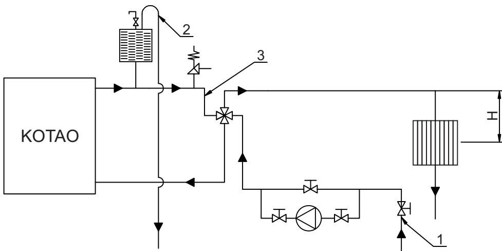
Slika 6.1 - sa četvorokrakim mešnim ventilom
