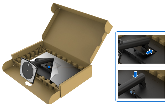
Slika 17. Umetnite jezičke na stubu stalka u proreze
