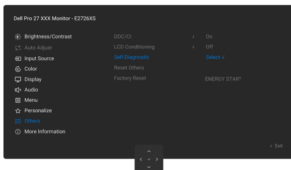
Slika 46. Ugrađena dijagnostika
