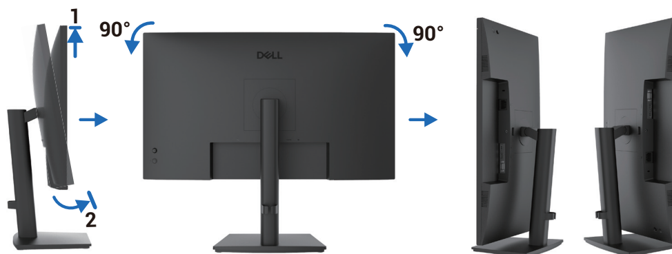
Slika 22. Rotiranje ekrana
