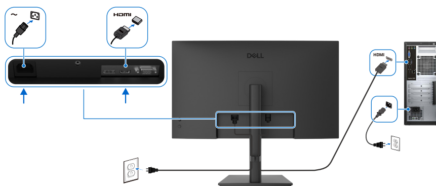
Slika 24. Priključivanje HDMI kabla
