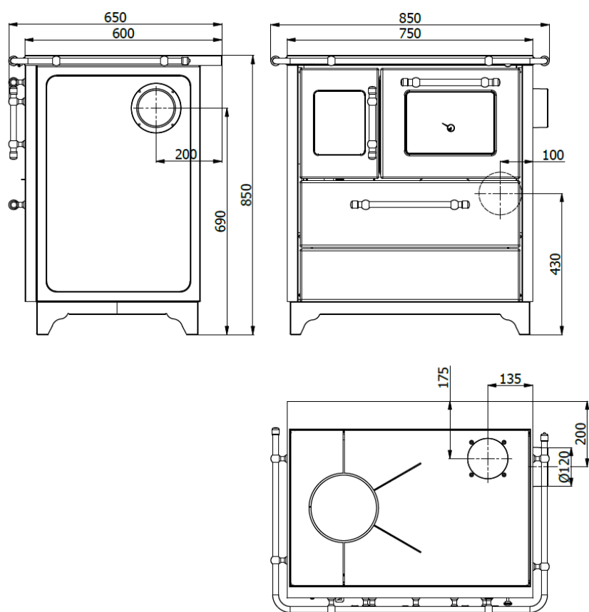
Slika 5 - DONNA 75- Dimenzije
