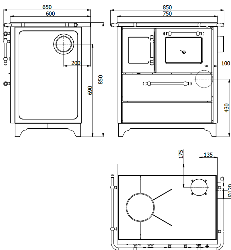
Slika 5 - DONNA 75- Dimenzije
