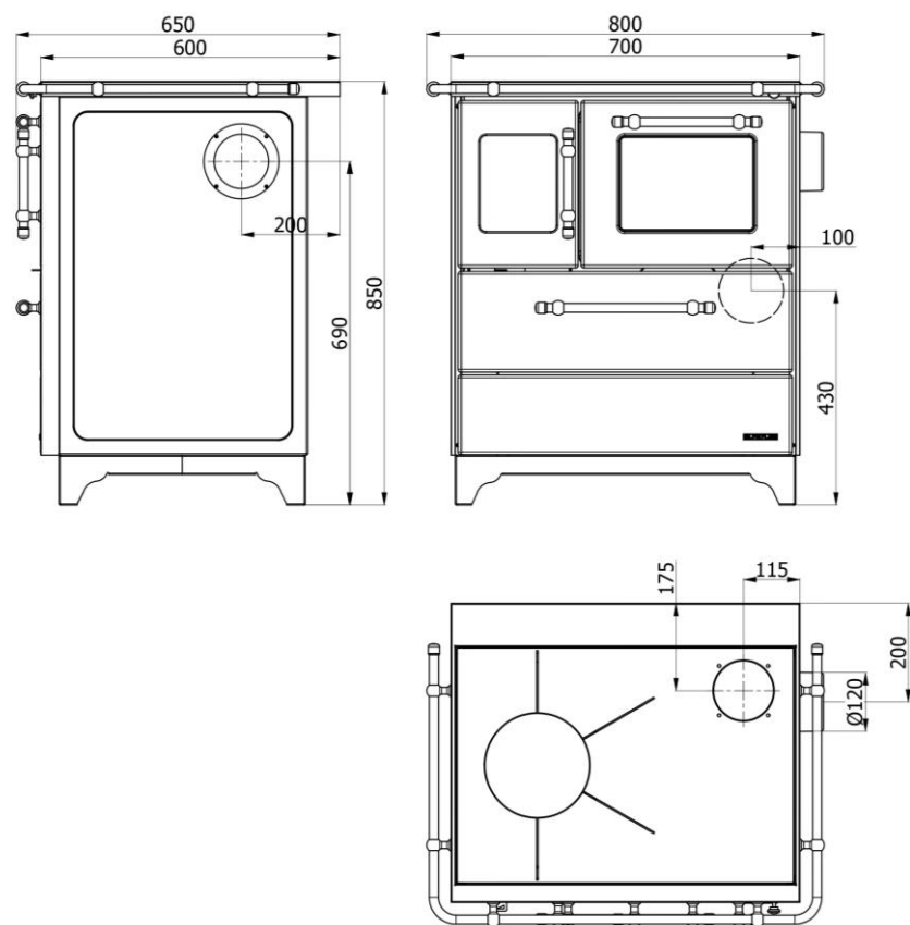
Slika 4 - DONNA70 - Dimenzije
