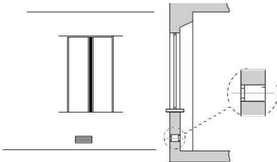
Slika 2.1: Primer neophodnog otvora za vazduh
