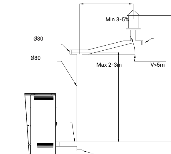
Slika 2.3: Izduvni kanal
