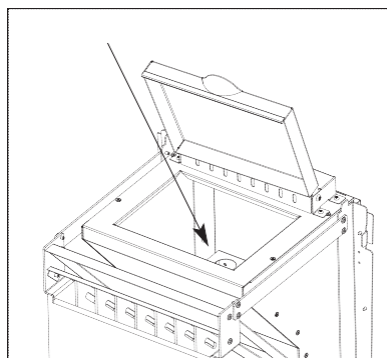
Ubacivanje peleta
