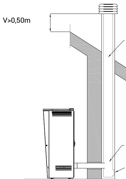
Slika 2.5: Odvod dima ka krovu putem tradicionalnog odžaka
