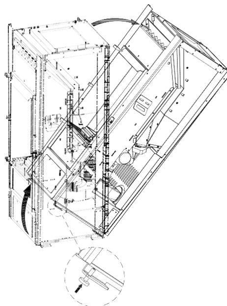
Slika 2.2.b: Nakrivljena peć
