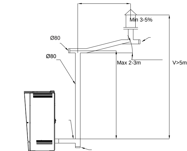
Slika 2.3: Izduvni kanal
