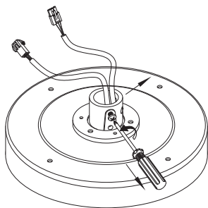
1. Popustite šaraf
