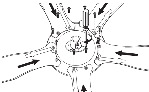
11. Šarafima pričvrstite lopatice za kućište motora
