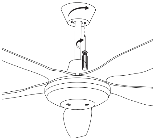
18. Fiksirajte dekorativni poklopac šarafima.
