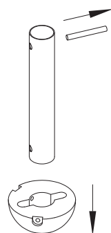
4. Izvucite osigurač
