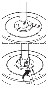
2. Izvucite osigurač iz poluge i izvucite polugu 3. Popustite šarafe
