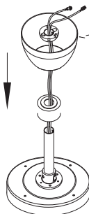
8. Provucite žice kroz dekorativni poklopac 9. Provucite žice kroz viseću kuglu 10. Fiksirajte viseću kuglu prema koracima 1, 2 i 3
