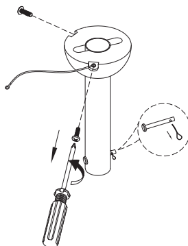
2. Izvucite osigurač iz poluge i izvucite polugu 3. Popustite šarafe
