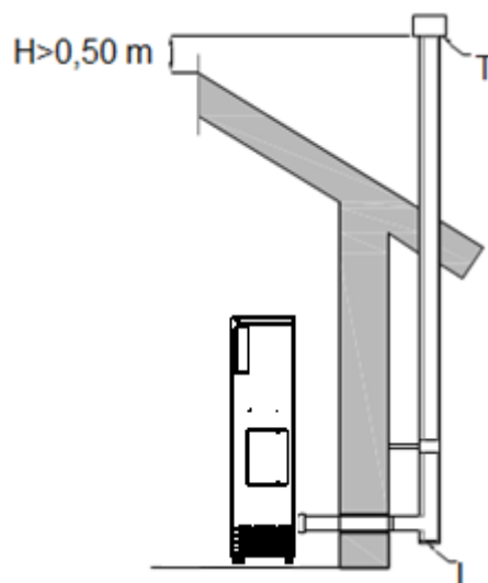
Slika 6.5: Odvod dima ka krovu putem tradicionalnog odžaka
