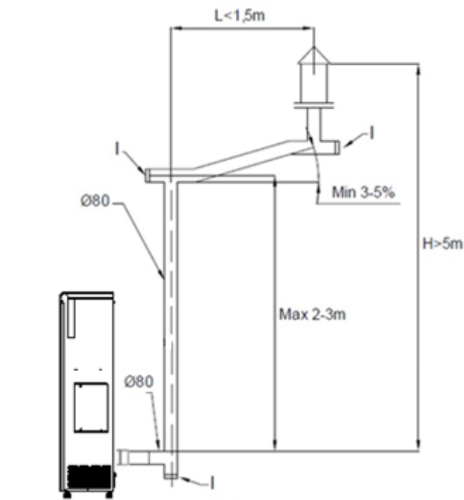
Slika 6.3: Izduvni kanal
