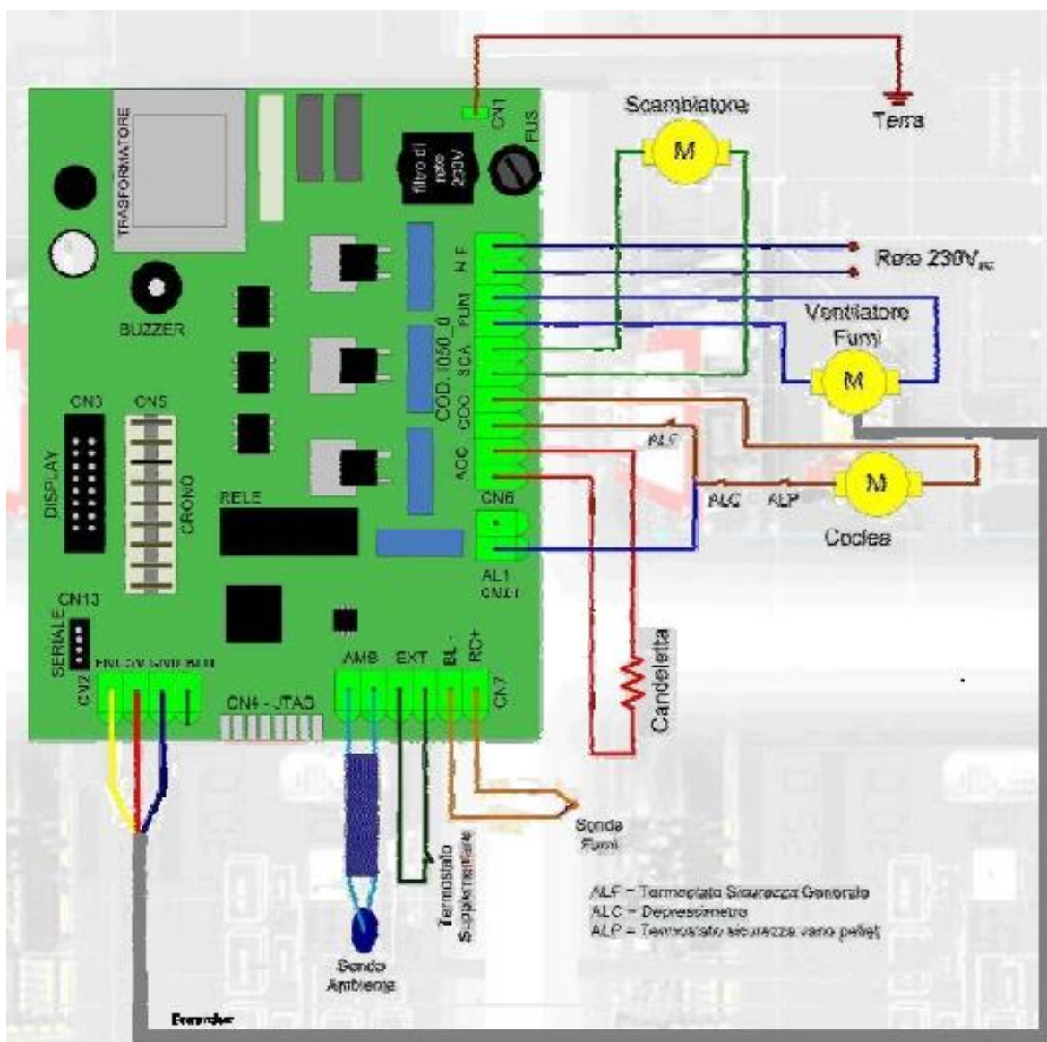
Slika 8.17. Elektronska kartica
