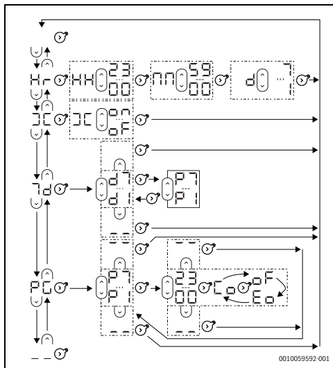
Fig. 3 Organigramme du menu des réglages de l'appareil
