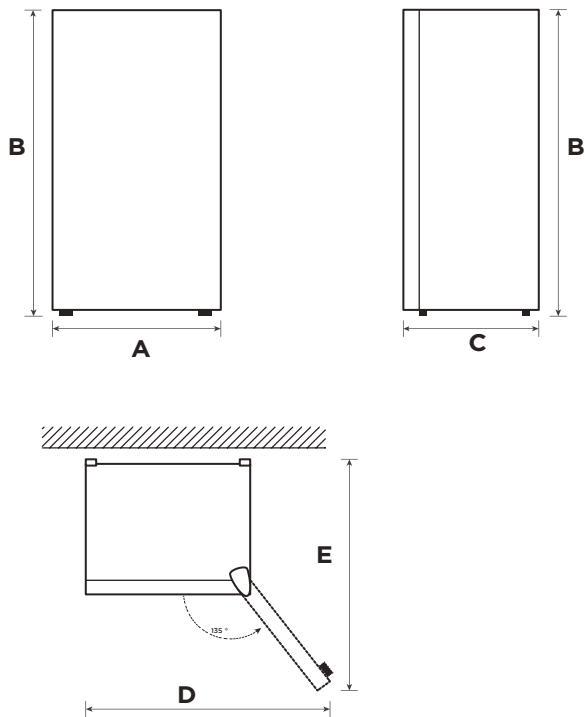
Diagrama spațiului necesar (când ușa este deschisă și când ușa este închisă)
