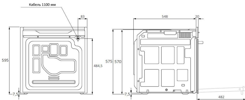
Вид ззаду
