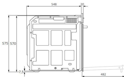
Sivusuunnasta
