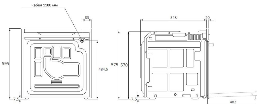
Изглед отзад
