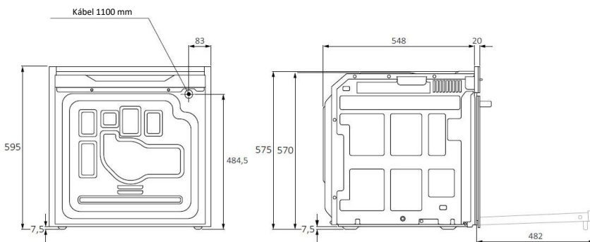
Hátsó nézet
