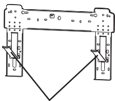
Ξεδιπλώστε τον βραχίονα της πλάκας τοποθέτησης
