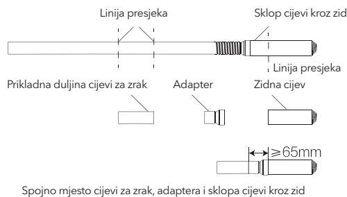
Spojno mjesto cijevi za zrak, adaptera i sklopa cijevi kroz zid
