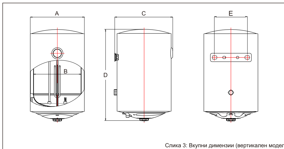
Слика 3: Вкупни димензии (вертикален модел)
