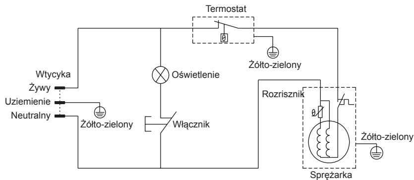
Schemat podłączenia
