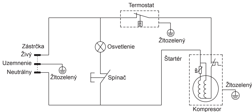
Schéma pripojenia
