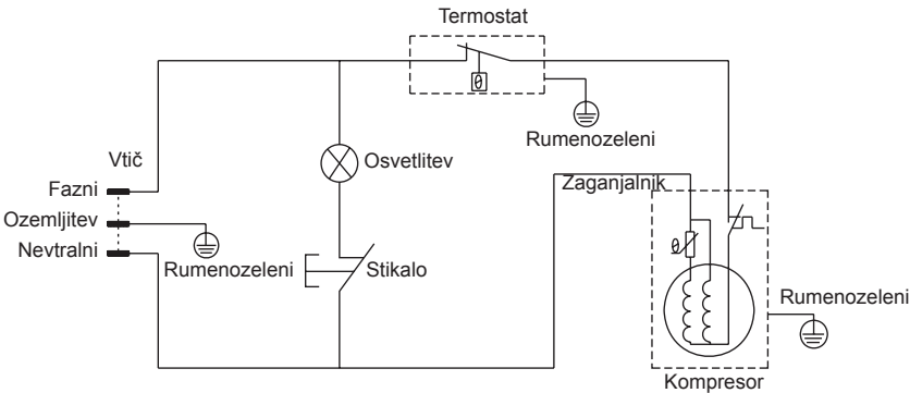
Shema priključitve
