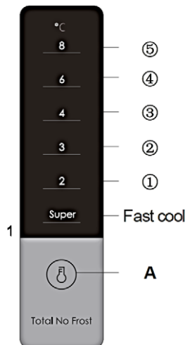
1B: Kontrola temperature na vratima frižidera (CF-310EDNF X)
