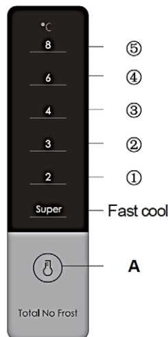
1B: Nadzor temperature na vratih hladilnika (CF-310EDNF X)
