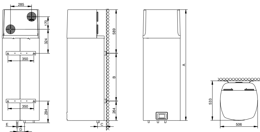
Slika 2: Priklučne i montažne mere toplotne pumpe (mm)
