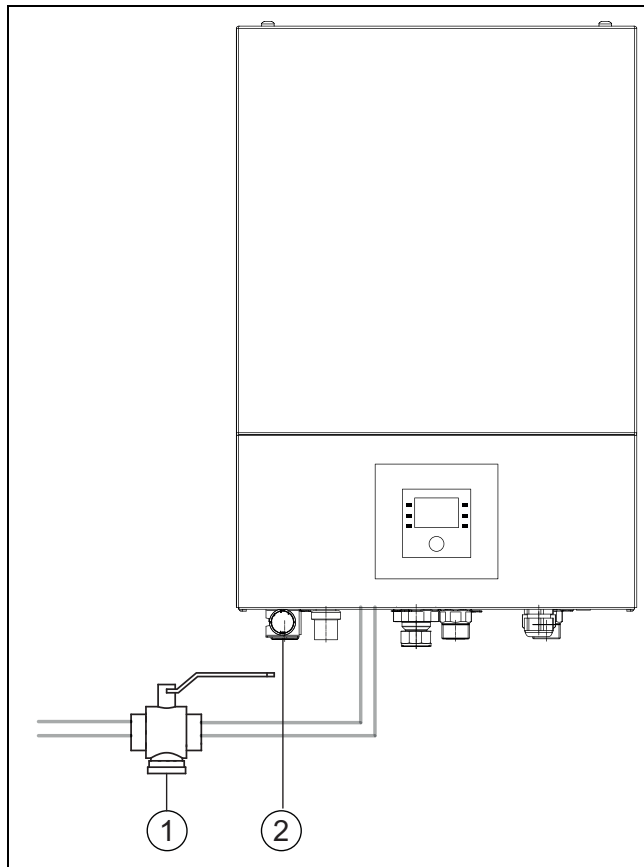
sl. 6 Unutrašnja jedinica AWE
