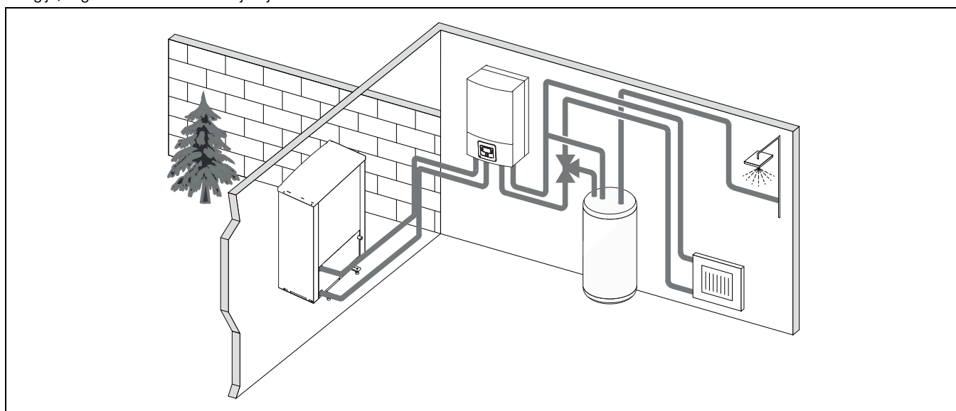
sl. 3 Toplotna pumpa Compress 6000 AW, unutrašnja jedinica AWE sa električnim dogrevačem i eksternim bojlerom za toplu vodu
