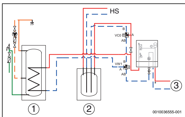
sl. 28 Bafer, VC0-ventil za premošćenje
