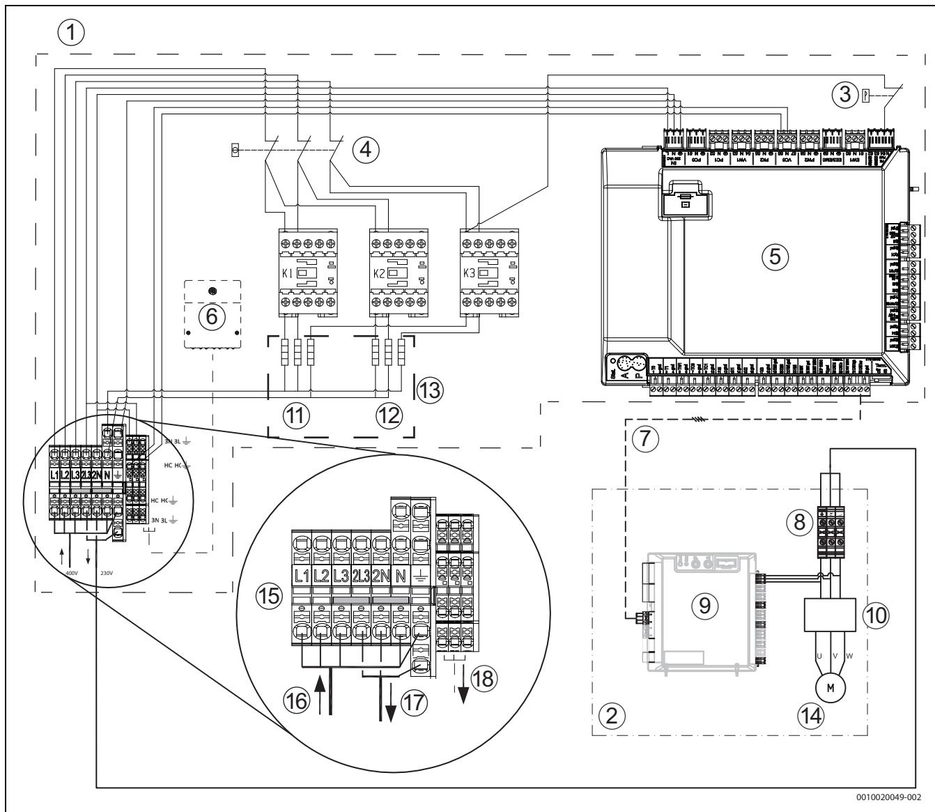
sl. 33 Jednofazna toplotna pumpa sa integrisanim električnim dogrevačem (trofazna struja)
