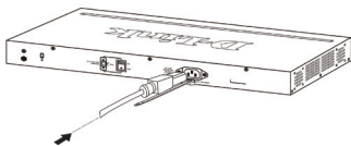
スイッチにAC電源ケーブルを挿入する
