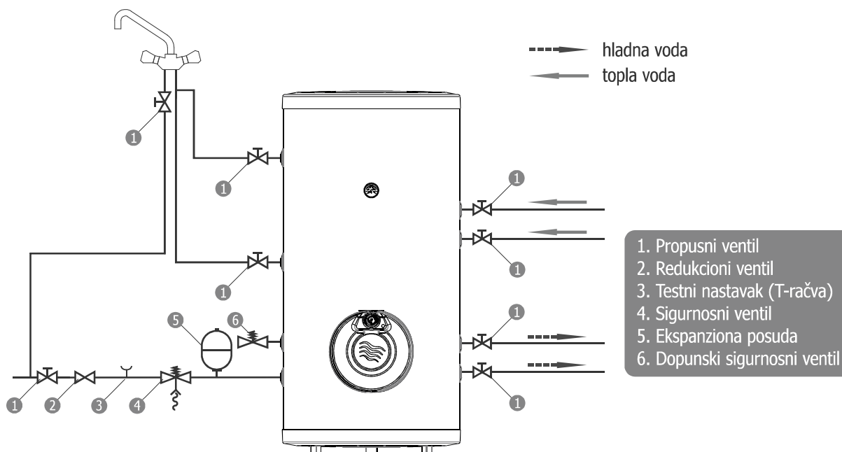
sl.2 Montažni crtež
