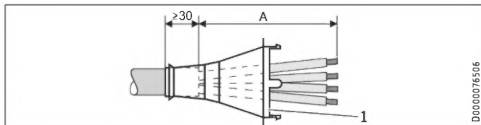
1 Kabeltülle
