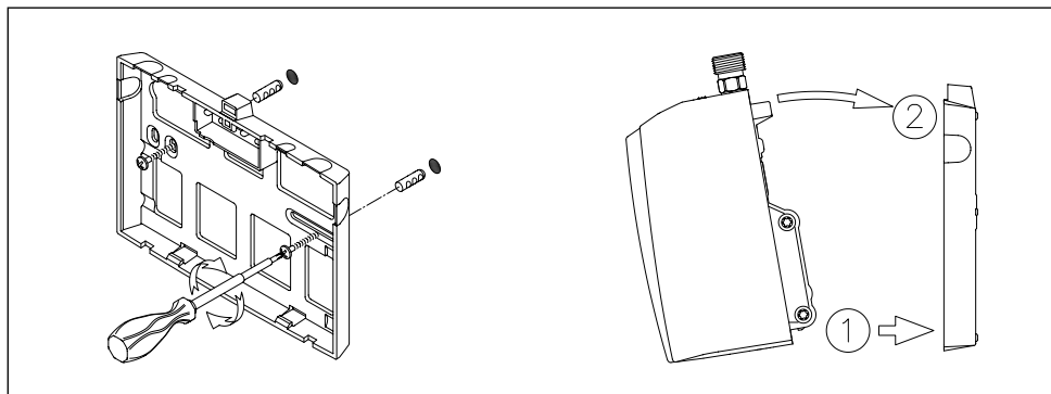
Абр. 4: "Монтаж на устройството за стена"
