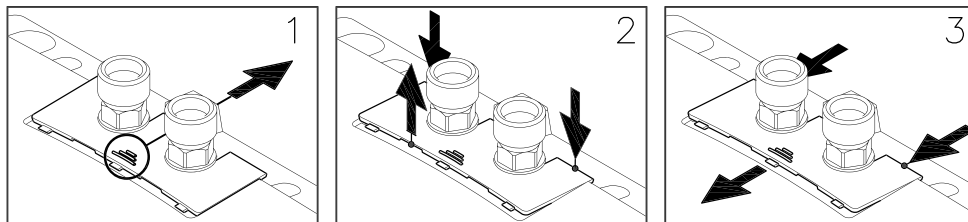
Obr. 9: »Demontáž krytu«
