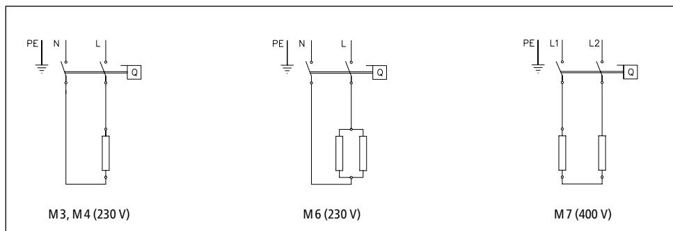
Fig. 6: «Koblingsskjema»
