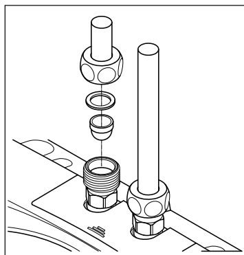
Abb. 12: »Wechsel des Filtersiebes«
