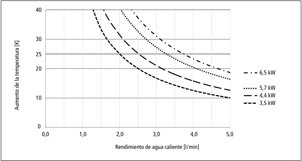
Fig. 11: «Aumento de temperatura y rendimiento de agua caliente»
