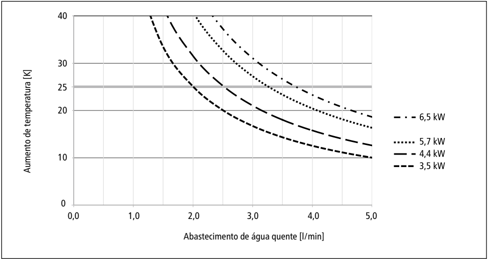
Ilustração 11: »Aumento da temperatura e abastecimento de água quente«
