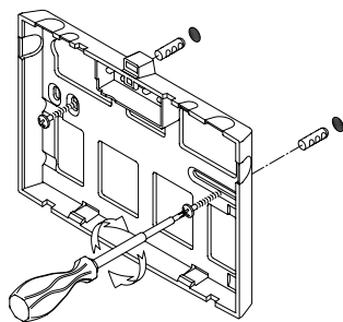
Rys. 4: »Montaż uchwyty ścienne«
