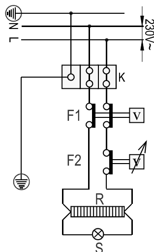
Elektro šema
