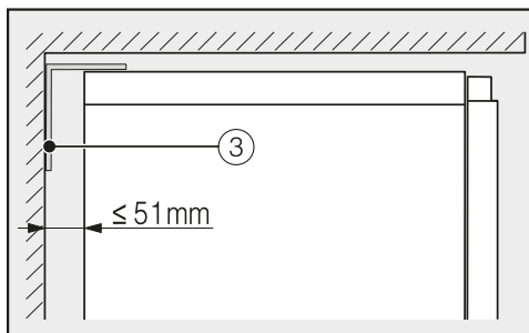
Pričvršćivanje za betonski zid
