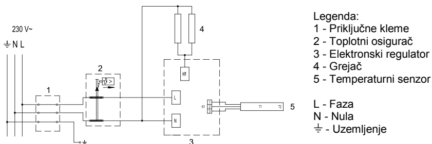
SI. 6: Šema povezivanja električnih provodnika
