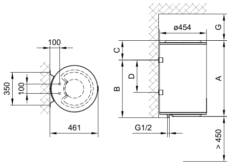
Fig. 1: Montimi vertikal në mur
