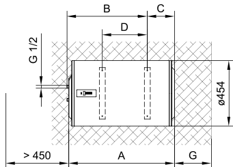
Sl. 2: Vodoravno postavljanje na zid
