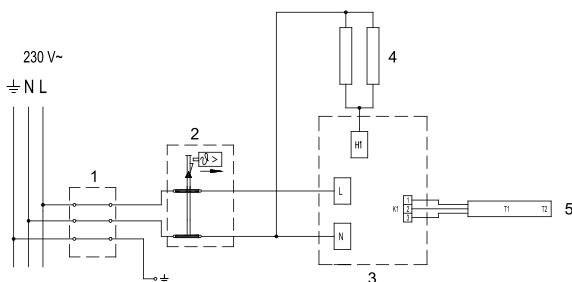
SI. 6: Električna spojna shema
