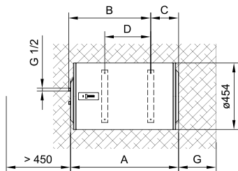
Sl. 2: Horizontalno postavljanje na zid
