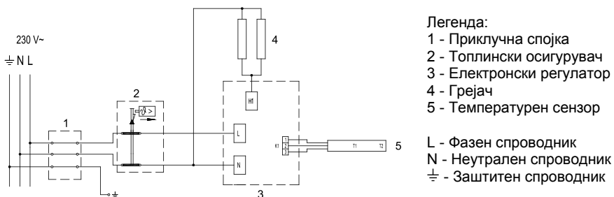
Слика 6: Шема на електрично поврзување
