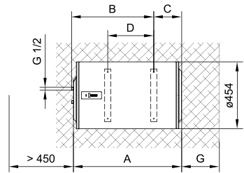
Abb. 2: Waagerechte Montage an die Wand
