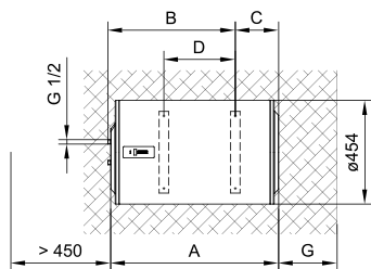
Sl. 2: Vodoravna namestitev na steno
