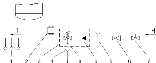
Fig. 3: Sistemi i mbyllur (me presion)
