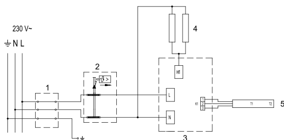
Fig. 6: Skema e lidhjes elektrike
