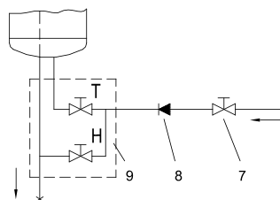
Fig. 4: Sistemi i hapur (pa presion)
