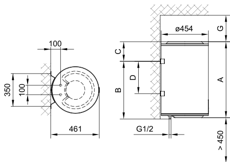
Sl. 1: Uspravno postavljanje na zid
