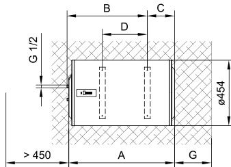
Fig. 2: Montimi horizontal në mur
