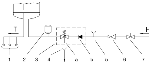
Abb. 3: Geschlossenes System (druckfestes System)
