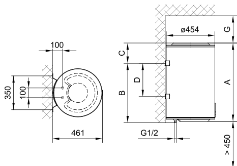
Sl. 1: Pokončna namestitev na steno
