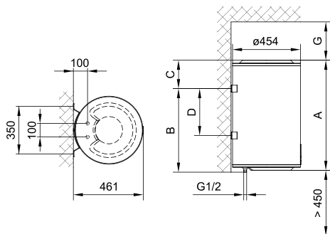
Сл. 1: Исправено поставување на сид
