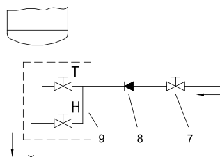
Sl. 4: Otvoreni sistem (protoćni)
