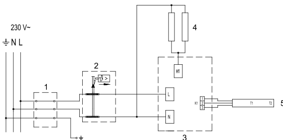
Abb. 6: Elektroschaltbild
