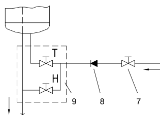
Sl. 4: Odprti (netlačni) sistem
