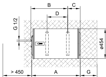
Сл. 2: Хоризонтално поставување на сид
