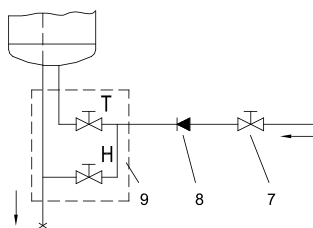
Sl. 4: Otvoreni (protočni) sustav
