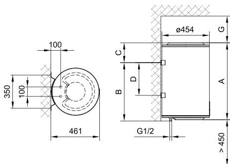
Sl. 1: Vertikalno montiranje na zid
