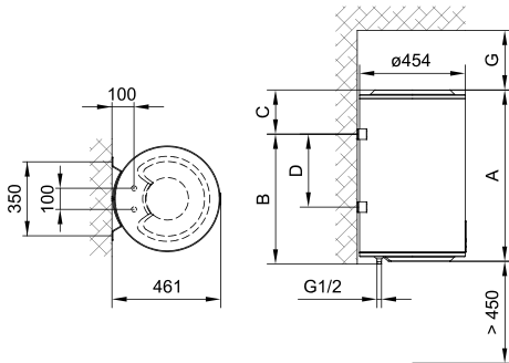
Abb. 1: Senkrechte Montage an die Wand
