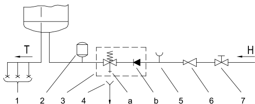
Слика 3: Затворен систем (со притисок)
