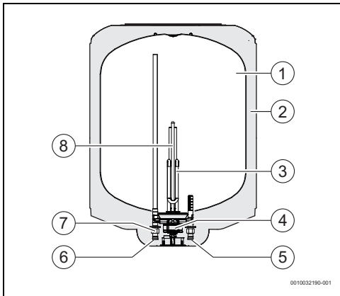
Fig. 3 Componentele aparatului
