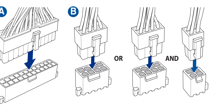
تثبيت توصيلات الطاقة ATX رابط های برق ATX را نصب کنید
