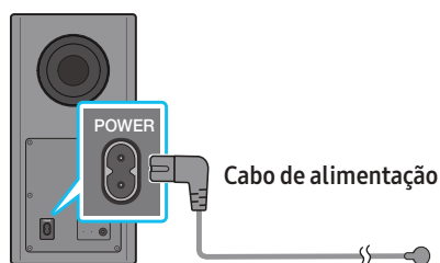
Parte de trás do Subwoofer
