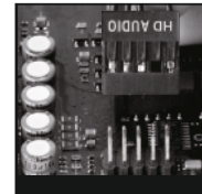
Auf richtige Polung achten Take care of correct polarity
