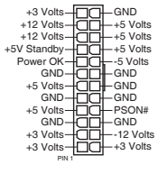
C ATX_PWR
