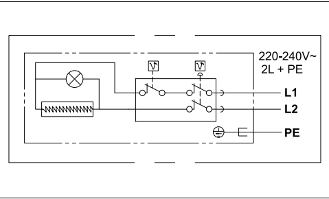
sl. 6 Shema priključivanja
