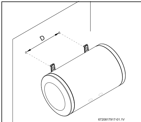
sl. 9 Horizontalna montaža (zidna montaža)
