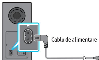
Spatele subwoofer-ului
