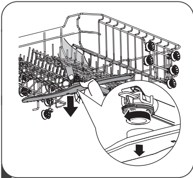
1 Da odstranite zgornjo pršilno roko, primate matico na sredini in jo držite na mestu, nato pa zavrtite pršilno roko v nasprotni smeri urnega kazalca, da jo odstranite.
