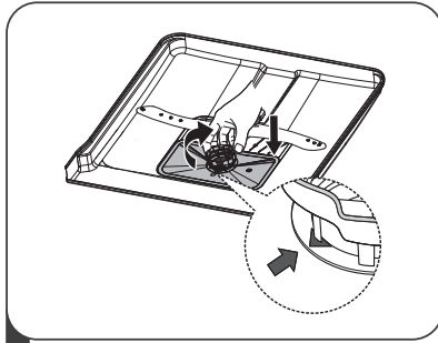
4 Filter znova sestavite po korakih, ki jih izvedete v nasprotnem vrstnem redu kot pri razstavljanju, znova namestite vložek filtra in obrnite v smeri urnega kazalca, ki jo kaže puščica.
