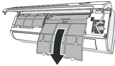
porvédő szűrő
