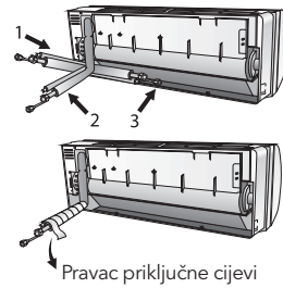
Pravac priključne cijevi
