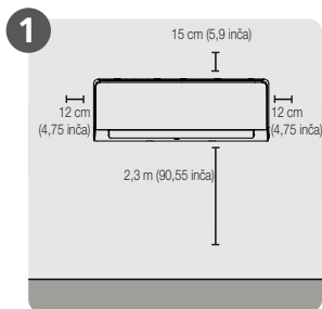
1 Odaberite mjesto ugradnje
