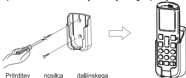
Pritrditev nosilca daljinskega upravljalnika
