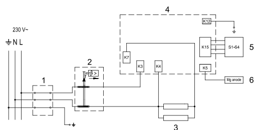
Električna spojna shema
