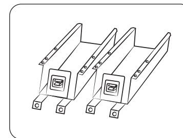
Consolă pentru partea inferioară (2)
