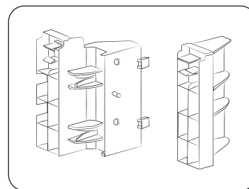
Držalo obrobe (2)
