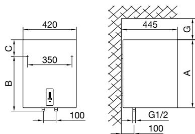
Fig. 1: Montimi vertikal në mur
