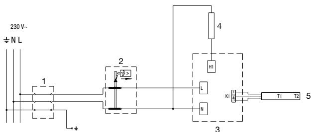
Sl. 5: Električna spojna shema
