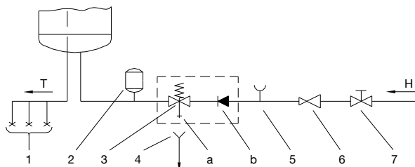
Sl. 2: Zaprti (tlačni) sistem
