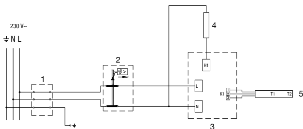
Сл. 5: Шема на електрично поврзување
