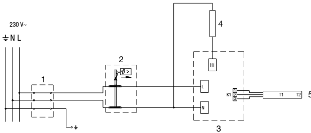
Bild 5: Elektroschaltbild
