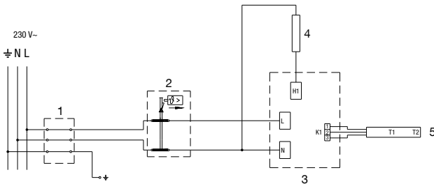
Sl. 5: Shema električne vezave
