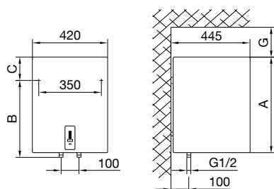
Sl. 1: Pokončna namestitev na steno
