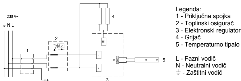
SI. 6: Električna spojna shema
