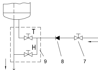
Слика 4: Отворен систем (прелевен)
