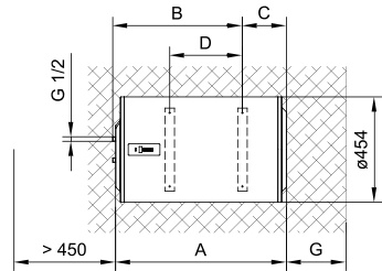
Fig. 2: Montimi horizontal në mur
