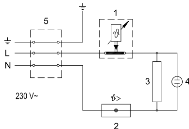
Schema električne vezave
